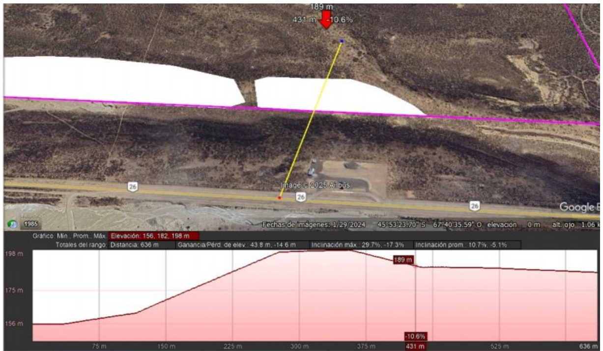
Figura 11: Sector 3 de explotación.
