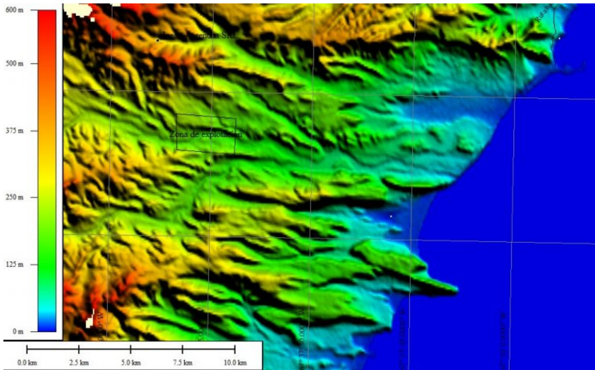
Figura 25. Mapa Topográfico 1. Imagen SRTM Global Mapper v16.1.
