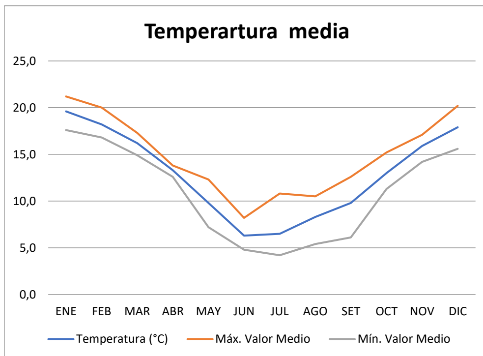
Figura 18. Temperaturas medias, máximas y mínimas en la ciudad de Comodoro Rivadavia para el período 1941/2022.
