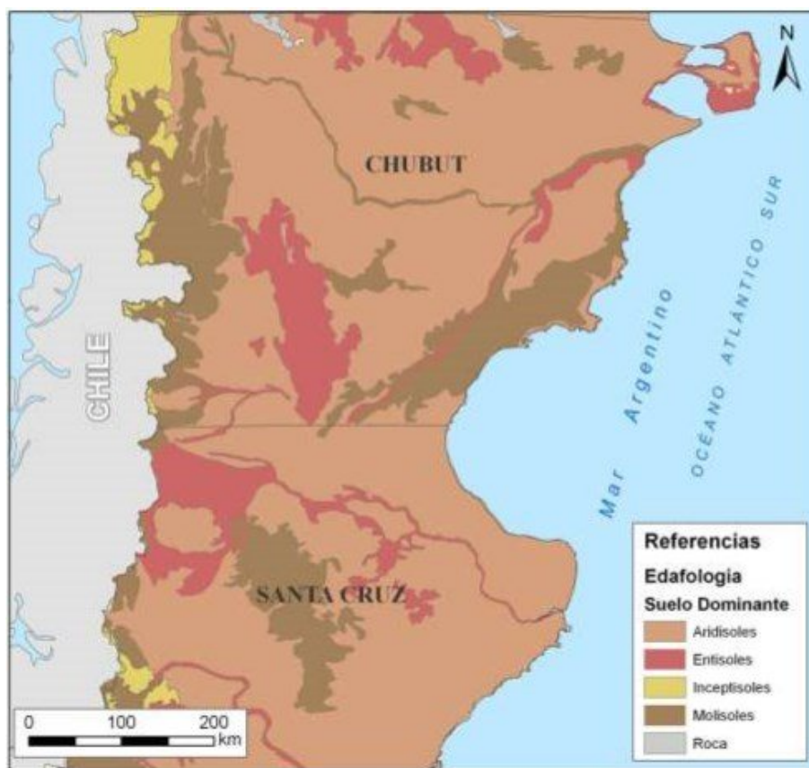
Figura 29. Mapa de clasificación de suelos (INTA).
