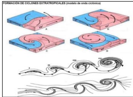
Figura 16. Modelo de formación de un ciclón.
