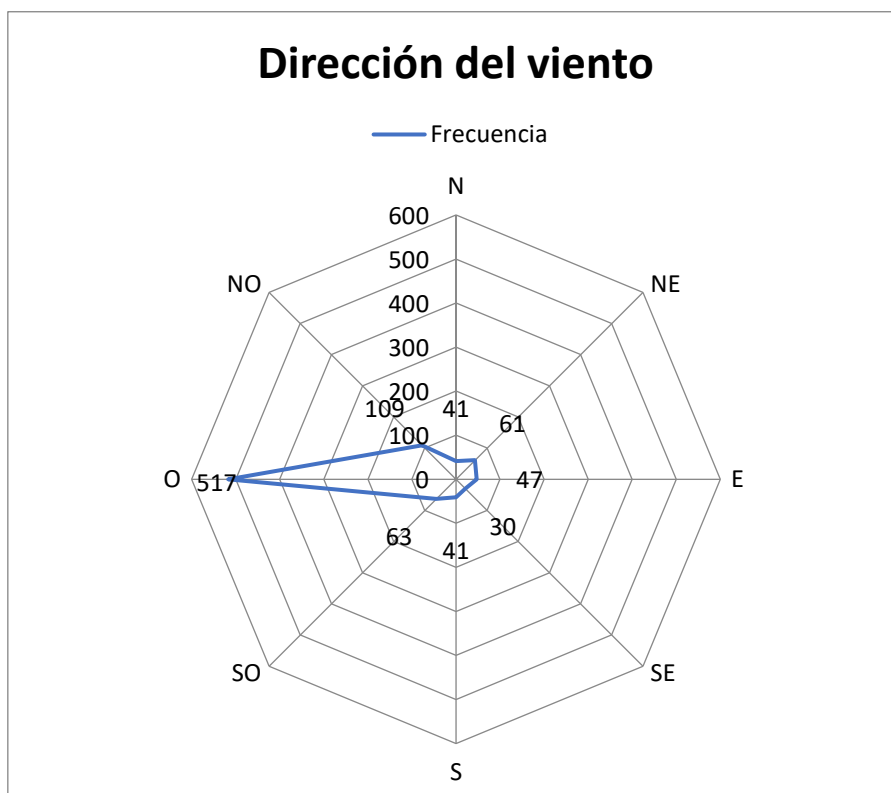
Figura 20. Direcciones de vientos predominantes.
