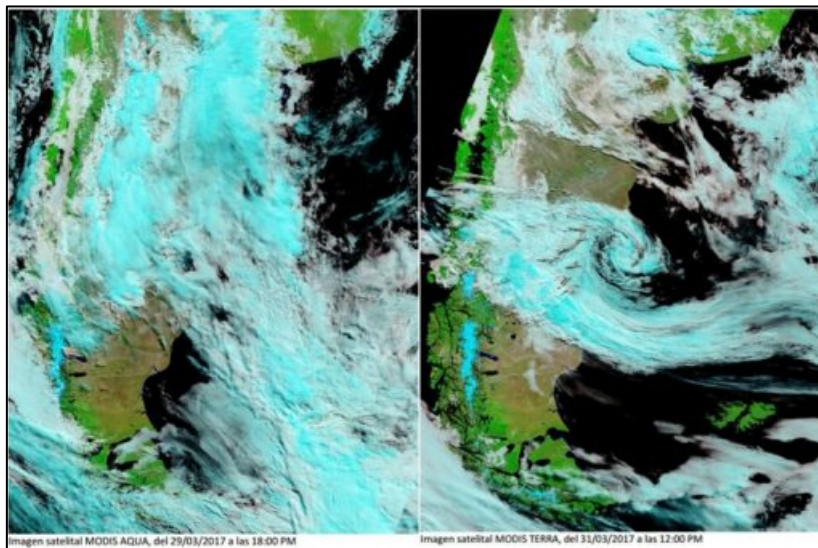
Figura 17. Imágenes satelitales de Modis Aqua de los días 29 y 31 de Marzo de 2017, donde se observa la nubosidad y generación del anticiclón extratropical.
