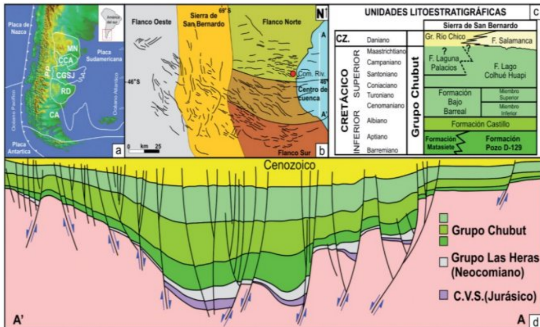
Figura 22. Tabla Tomada de Allard et al., 2015. a) Ubicación de la CGSJ (CA: Cuenca Austral, RD: Región del Deseado, CGSJ: Cuenca del Golfo San Jorge, CCA: Cuenca de Cañadón Asfalto, MN: Macizo Nordpatagónico, PP: Precordillera Patagónica). b) Dominios Estructurales (Figari et al. 1999), c) Unidades litoestratigráficas del Grupo Chubut (Casal et al. 2015). d) Corte estructural regional en el que se destaca la estratigrafía vinculada a la CGSJ para los depósitos Jurásicos-Cretácicos (Figari et al. 1999).
