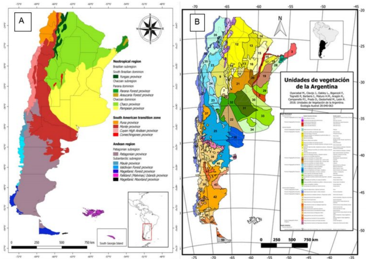
Figura 31. A- Mapa biogeográfico de Argentina (Arana et al. 2017); B- Unidades de vegetación de la Argentina agrupadas en provincias y ecotonos fitogeográficos, dominios y regiones. Se indican los nombres fisonómico-florísticos propuestos y los nombres populares o más conocidos (extraído de Oyarzabal et al. 2018).
