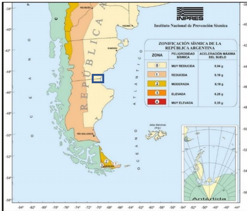
Figura 27. Mapa de zonificación Sísmica. INPRES.
